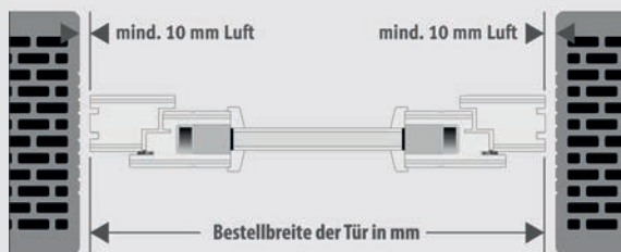
Breitenaufmaß in Laibung
