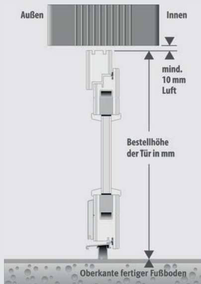
Höhenaufmaß in Laibung
