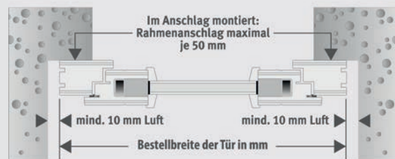
Breitenaufmaß mit Anschlag
