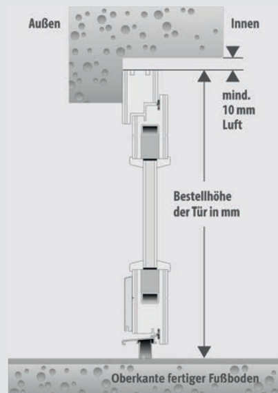
Höhenaufmaß mit Anschlag
